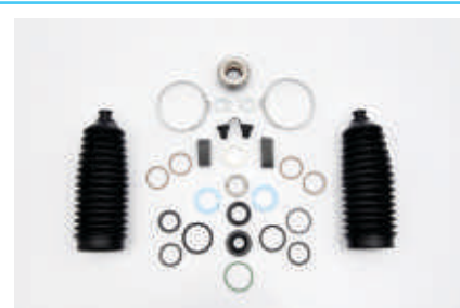
CX.33318 e CX.33318/2 (sem coifas)
