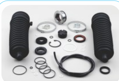
CX.33914 e CX.33914/2 (sem coifas)
